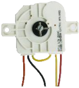
LE 15min 4wire
