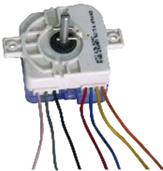
LBP 15min 7wire
