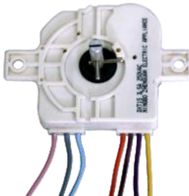
SS 15min 7wire
