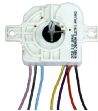
SS 35min 7wire
